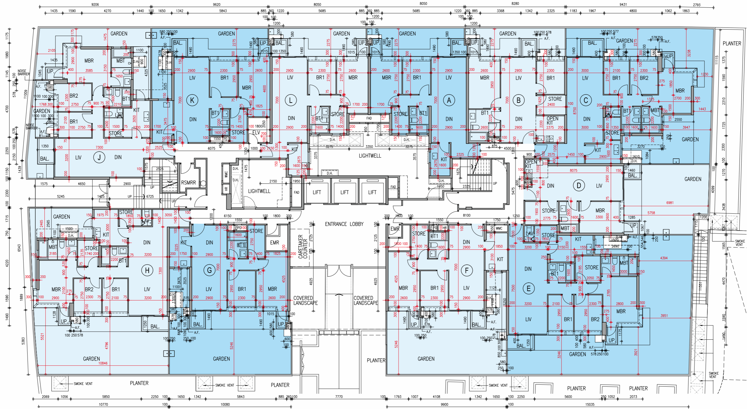
TOWER 1 第一座 GROUND FLOOR PLAN 地下平面圖
