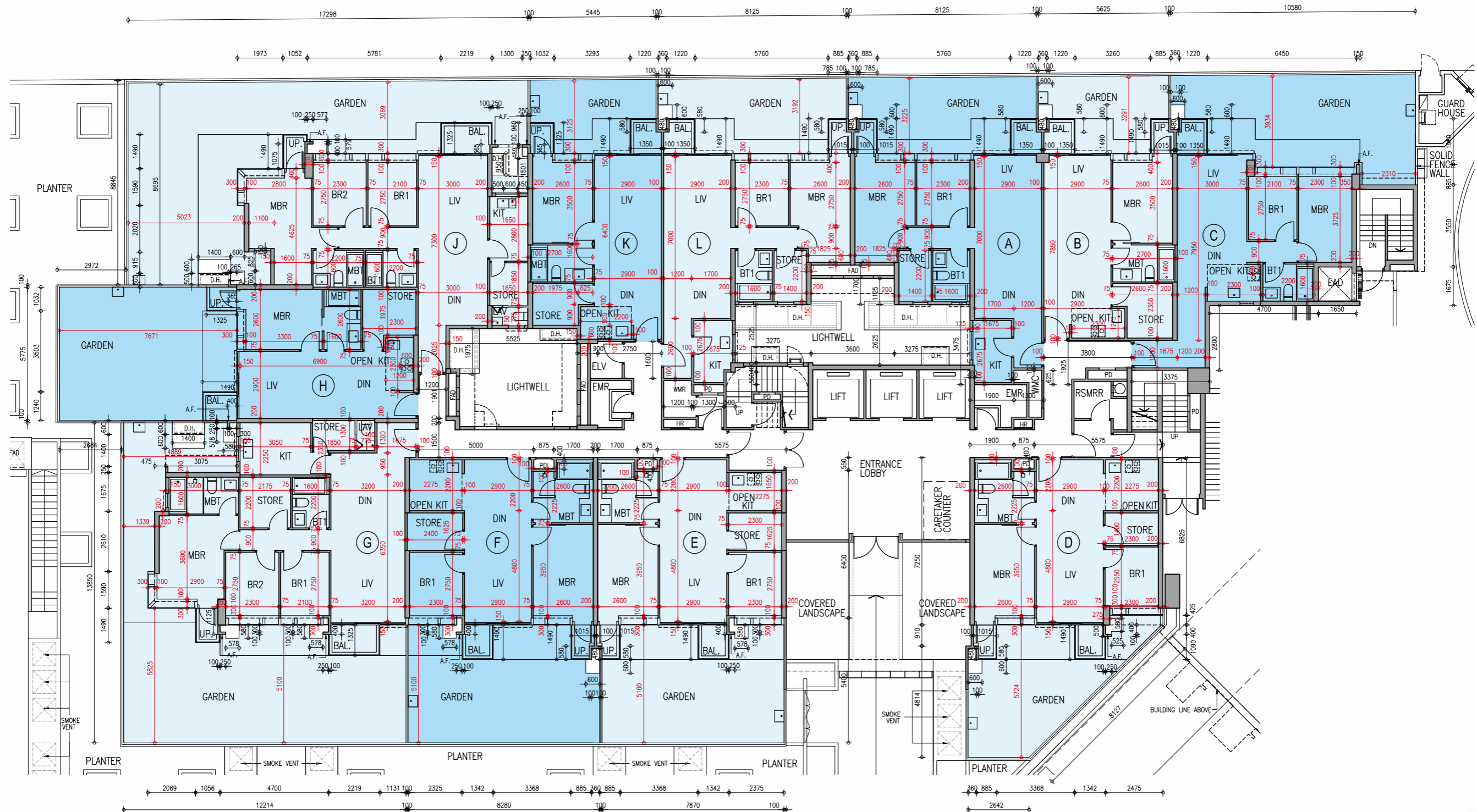
TOWER 2 第二座 GROUND FLOOR PLAN 地下平面圖
